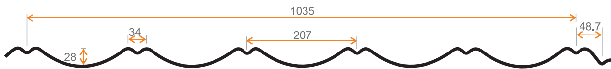
MEDIDAS (mm)
